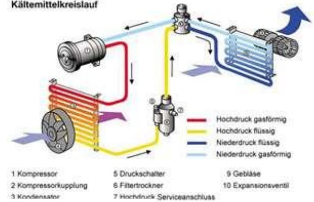
Kältemittelkreislauf
